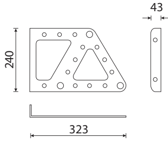
TAL-24 Staffa fissaggio parete in alluminio Wall aluminium bracket
