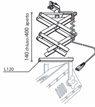
XTSAF-PP Finitura: alluminio zincato Finiture: galvanized aluminum
