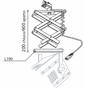
XTSAF-PG Finitura: alluminio zincato, nero e bianco Finiture: galvanized aluminum, black and white
